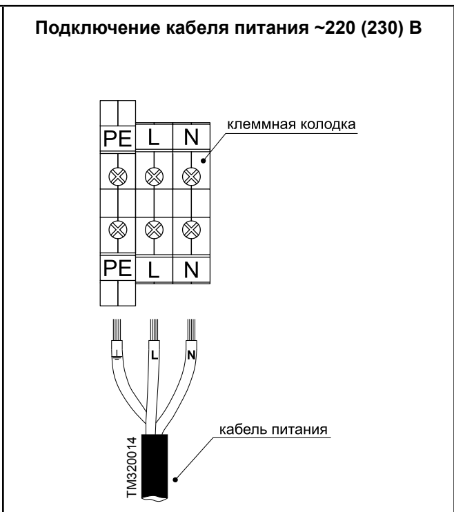
Схема подключения группы завес к однофазной сети переменного тока с напряжением ~220 (230) В
